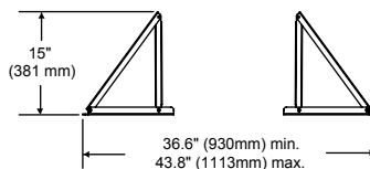
CM50(-S)
